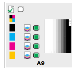
Prosessi valmis
