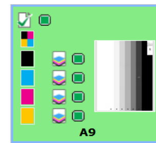
Sivu hyväksytty
