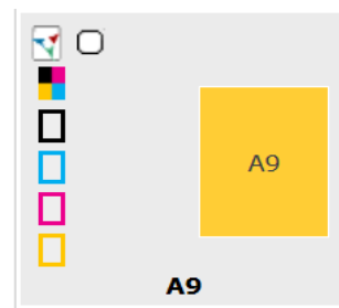
Sivu prosessoituu
